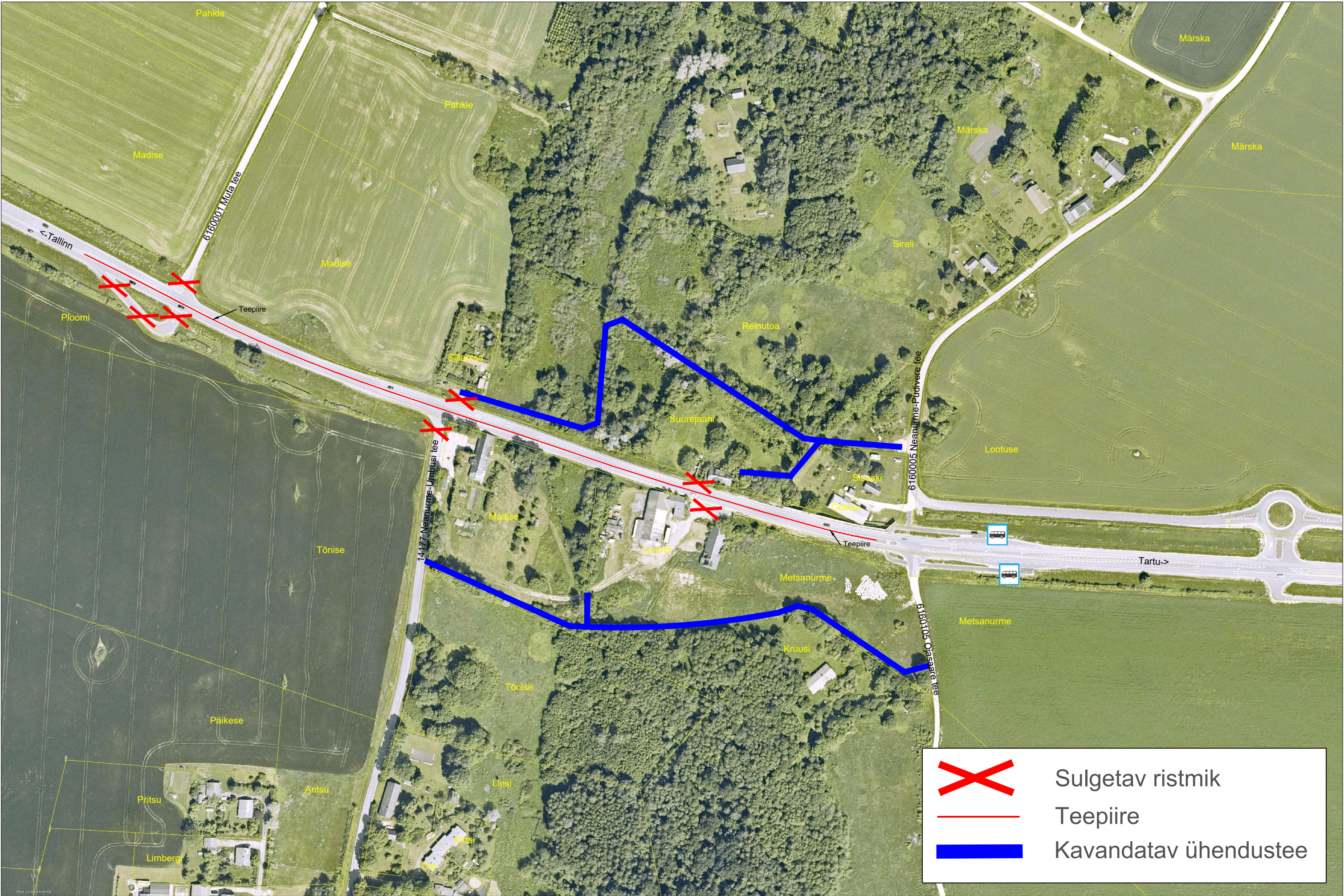
Lisa. Eskiisjoonis. Riigitee 2 Tallinna-Tartu-Võru-Luhamaa km 129,6-130,3 Neanurme küla liiklusohtliku koha likvideerimine
